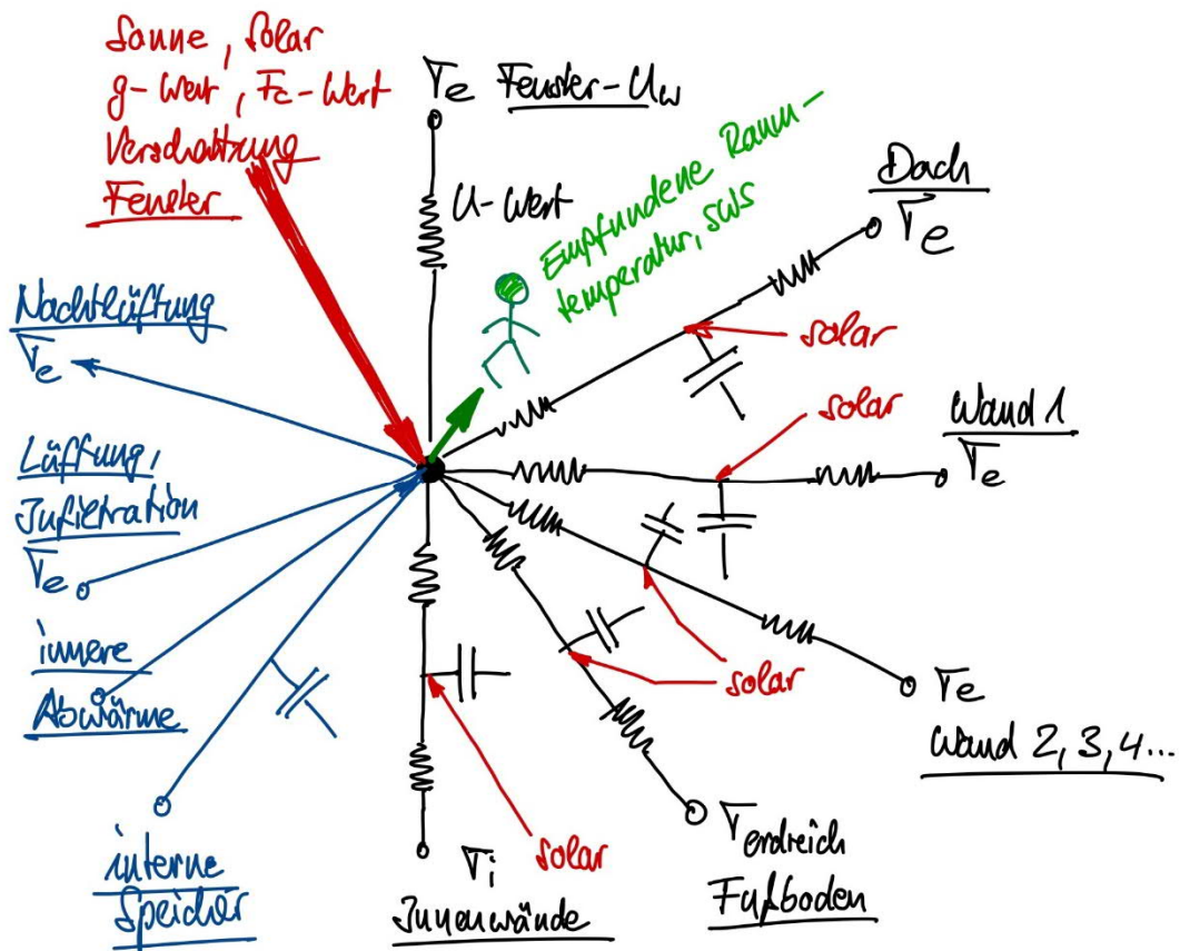
Bild 2: Prinzip „Schaltbild“ der Einflussgrößen auf die empfundene Raumtemperatur unter außenseitiger Hitzeeinwirkung und der Energiepfade, bestehend aus Temperaturnoten, Wärmedurchgangswiderständen und Wärmespeicherfähigkeiten. T e = Außenlufttemperatur, T i = Innenlufttemperatur.
